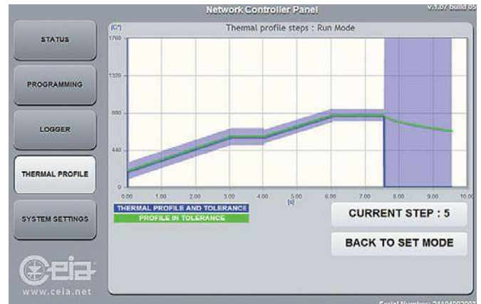
Bildschirmanzeige des Temperaturprofils in Echtzeit
